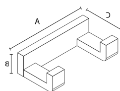
Cabide IL 9022 Material: Inox 304
