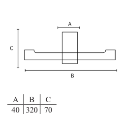
Papeleira Dupla Material: Latão / Vidro
