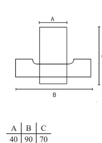
Cabide Material: Latão
