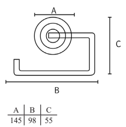
Papeleira Material: Latão
