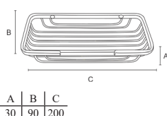
IL 9500 - Saboneteira Parede G Material: Latão
