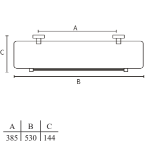
Porta Shampoo c/ Grade Material: Latão / Vidro
