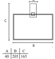
Porta Toalha Argola Material: Latão
