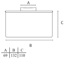
Papeleira Material: Latão
