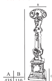
Castiçal - IL6304 Material: Ferro
