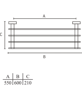
Porta Toalha Rack Material: Latão
