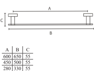
Porta Toalha Material: Latão
