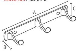
Cabide 9004-3 Material: Alumínio
