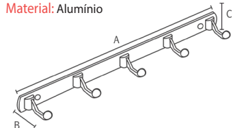
Cabide 9004-5 Material: Alumínio
