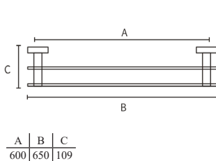
Porta Toalha Duplo Material: Latão
